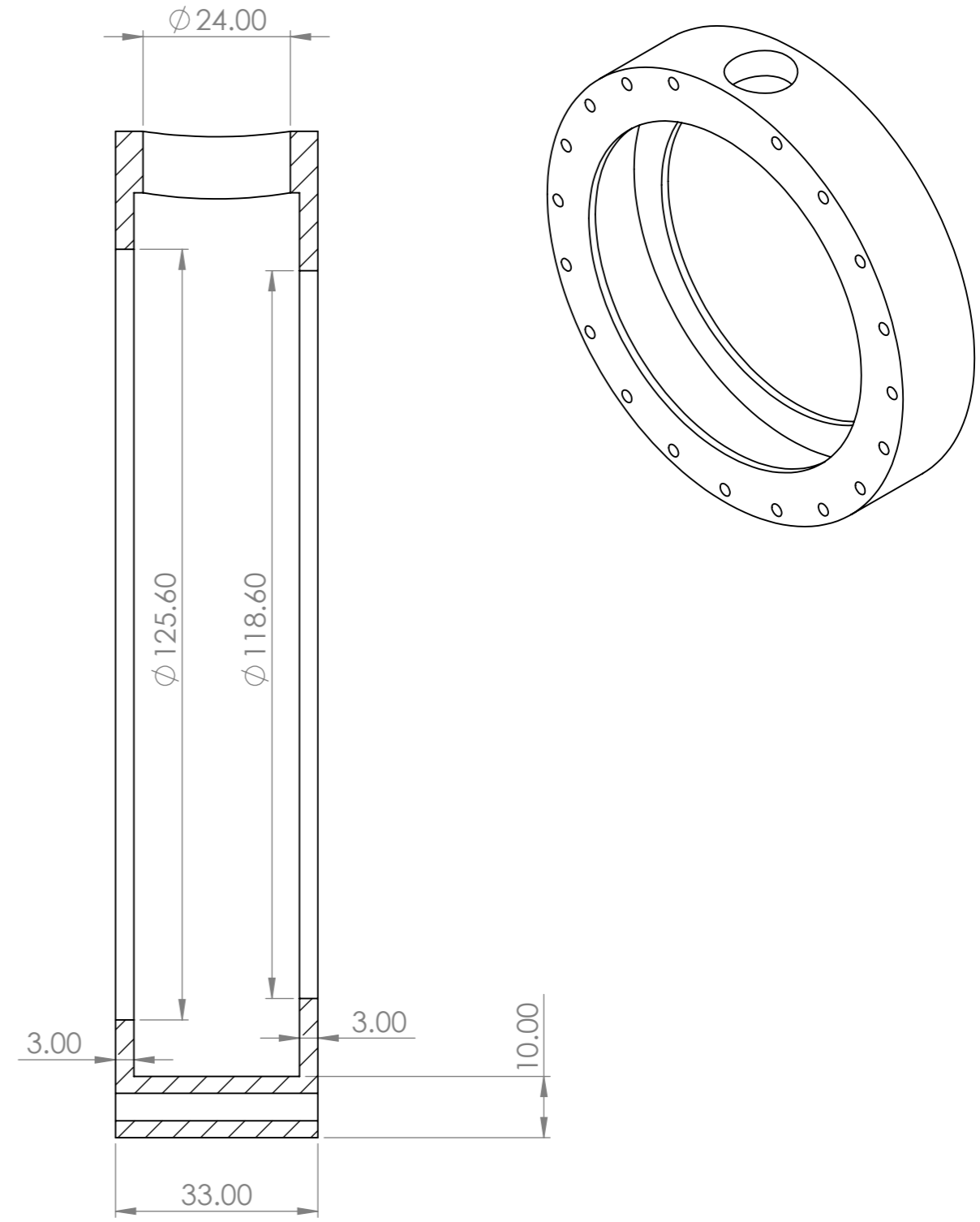
SECTION A-A
